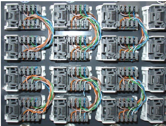
Figura 27 – Painel traseiro do secundário de um DDC
