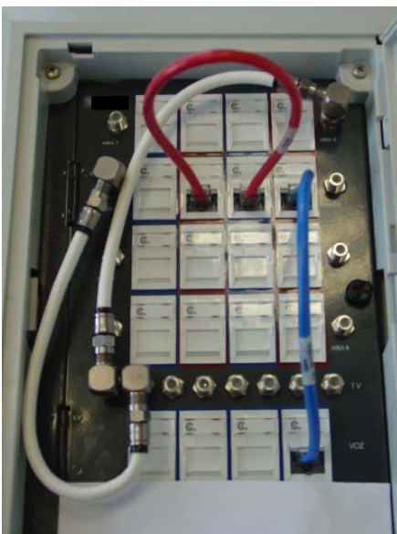
Figura 29 – ATI, exemplo de ligações de cliente
