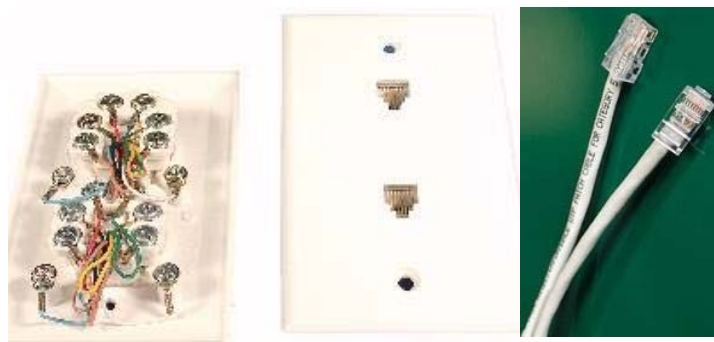
Figura 33- Tomada dupla de 8 contactos, vista pela frente e verso e respectivas fichas
