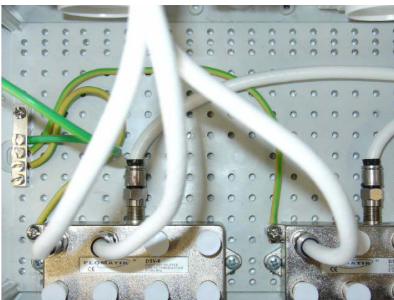
Figura 31 – Pormenor de ligações aos TC, num ATI
