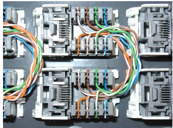
Figura 28 – Exemplo de um paralelo entre 2 tomadas RJ45
